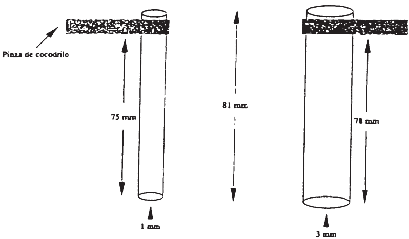
Dimensiones de los electrodos
