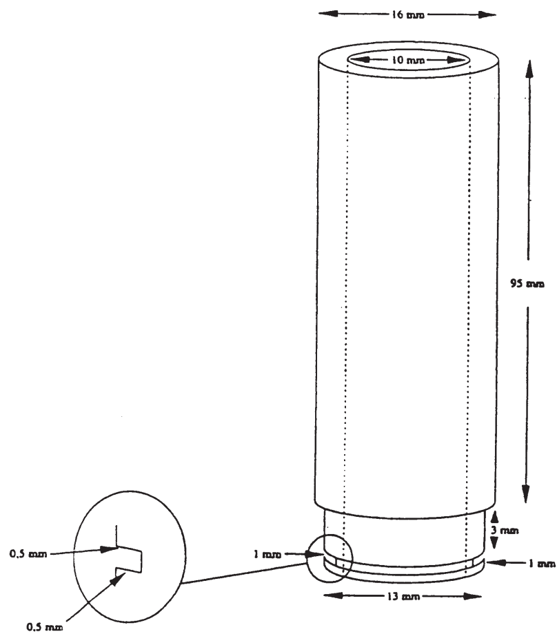
Figura 1 Dimensiones del tubo de PTFE
